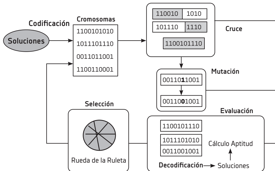
Esquema básico de un algoritmo genético. (Parra Trujol, 2013)
