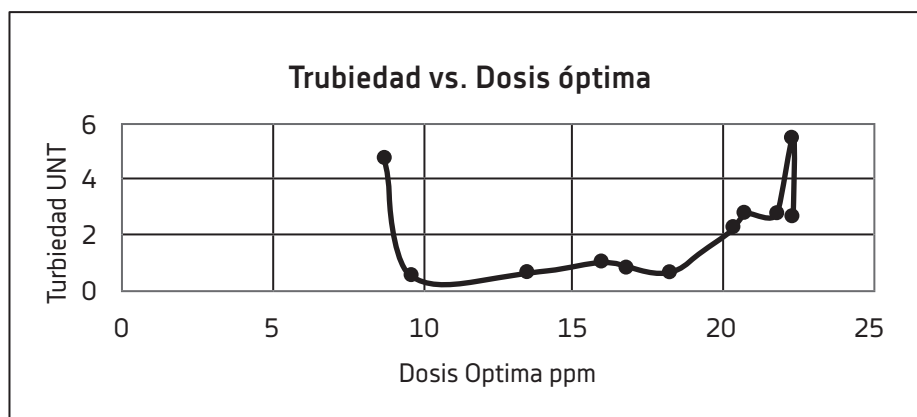
Turbiedad (UNT) vs. dosis optima ppm.
